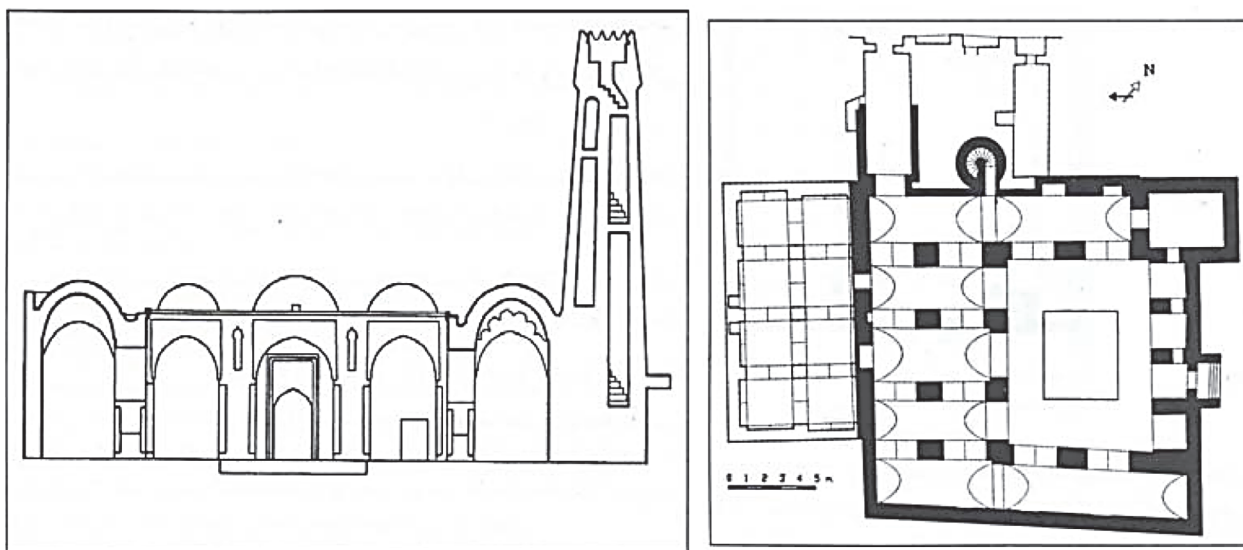
شکل ۱. پلان و برش بنای مسجد فهرج (انیسی، ۱۳۸۹)
