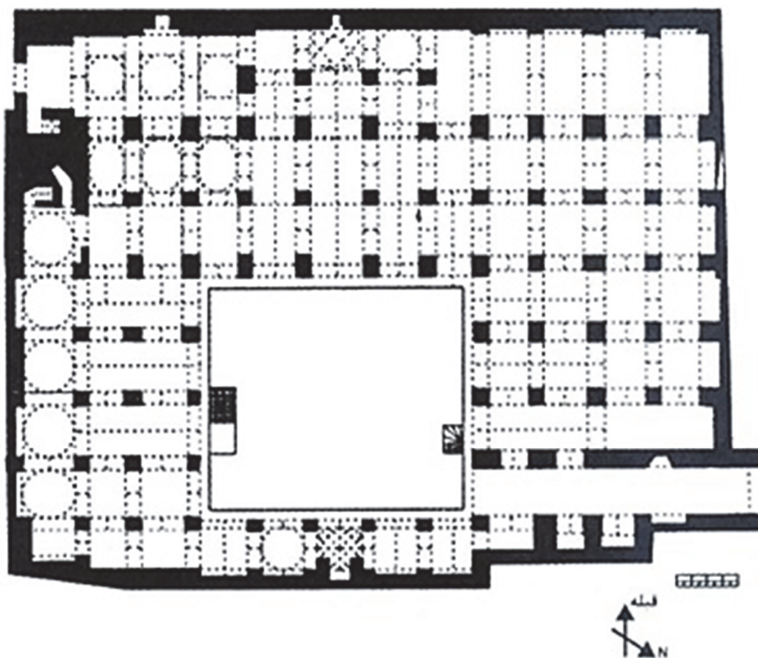
شکل ۷. پلان مسجد جامع نایین (تجلیل، ۱۳۹۸)
